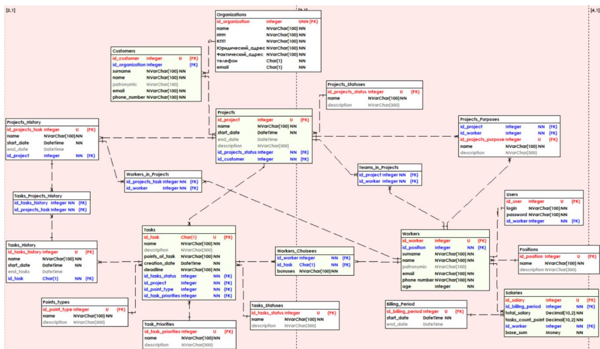
Рис 3 - Физическая модель приложения
