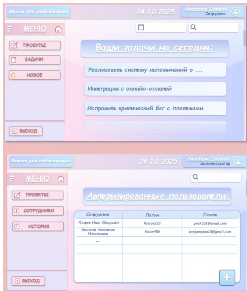
Рис. 4 - Страница Меню для: Сотрудников/Тимлидов и Администраторов
