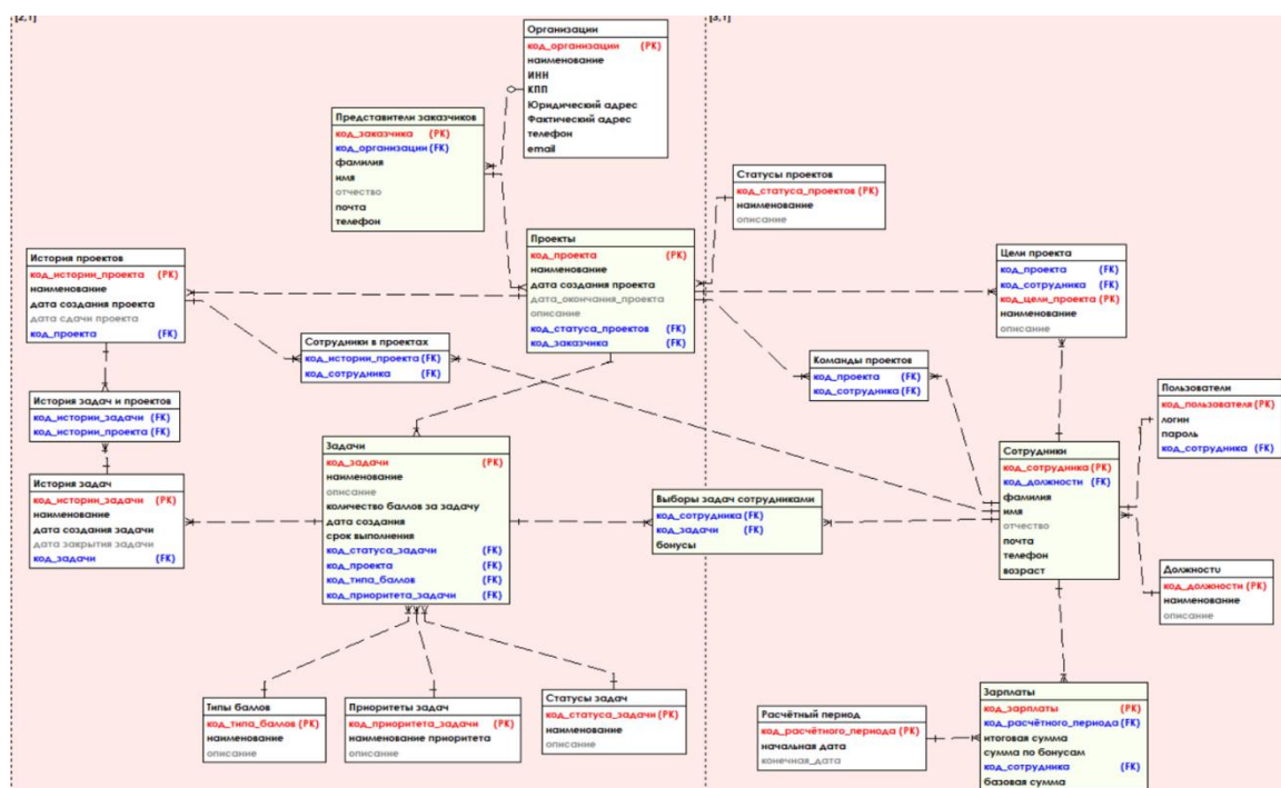
Рис 2 - Логическая модель приложения
